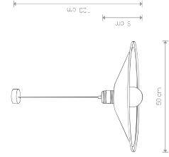
GARRET
